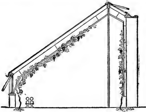
FIG. 97. FORCING GRAPERIE ( Section ).
